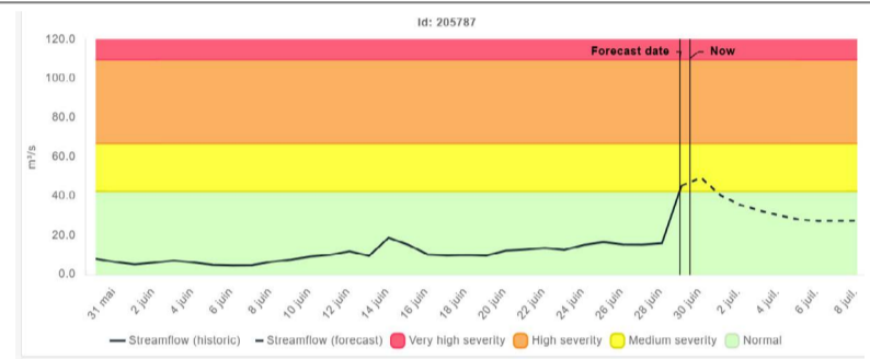
Figure 2 : Courbe de variation des débits à la station de Togblécopé (Zio)
