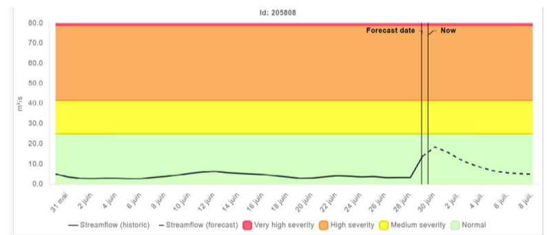
Figure 3 : Courbe de variation des débits à la station de Gati (Haho)
