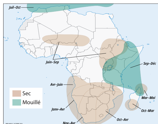
CARTE S1.2.1 Conditions météorologiques attendues liées à El Niño
